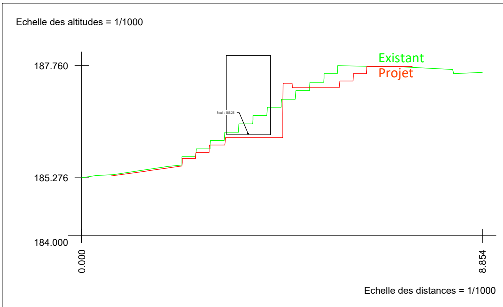
Coupe à l'axe de l'escalier existant
